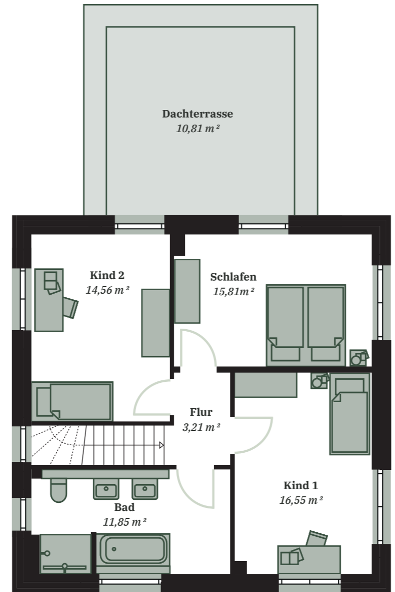
DACHGESCHOSS
